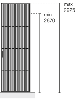
Pannello con tre traversi orizzontali. Panel with three horizontal crosspieces
