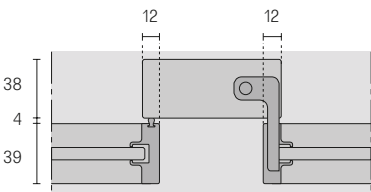
Sistema di scorrimento con trascinio Sliding system with connecting plate
