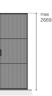
Pannello con due traversi orizzontali. Panel with two horizontal crosspieces
