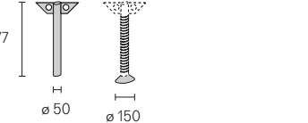
Gamba strutturale in metallo con e senza elica passacavi / Structural metal leg with and without spiral cable guide
