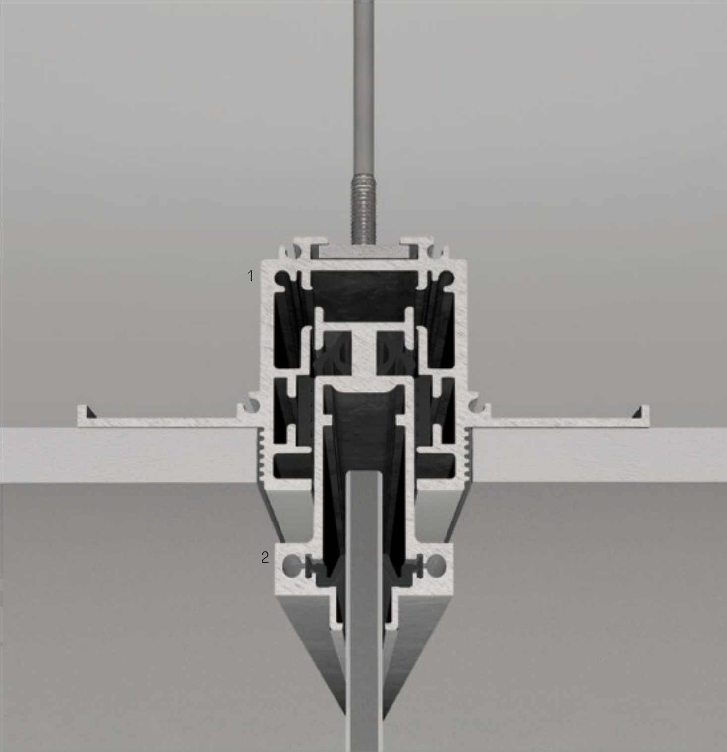
Profilo singolo incasso totale Single built in profile
