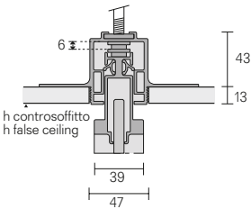
Profilo singolo incasso totale Single built in profile
