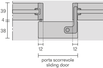
Sistema di scorrimento con trascin Sliding system with joint connection
