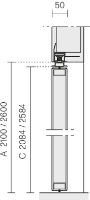
Porta battente filo parete Wall flush swing door
