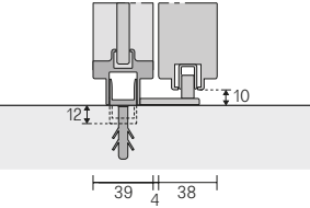
Sistema di fissaggio a terra con regolazione di 12 mm Floor fixing system with 12 mm adjustment
